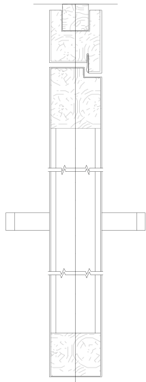
ABSC.S Sezione verticale sopraluce Fanlight vertical section
